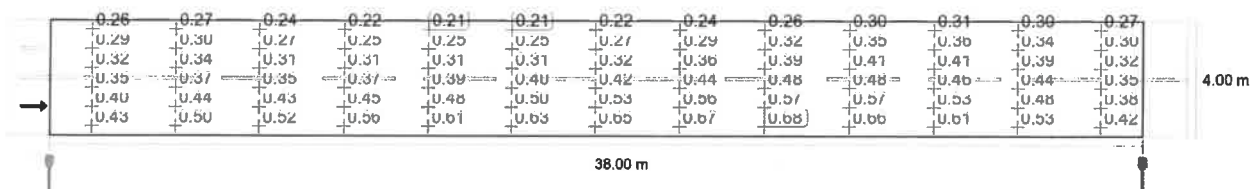
Observator 1: Valoarea de întreținere, densitatea luminii cu carosabil uscat [ \text{cd}/\text{m}^2 ] (Raster valoric)
